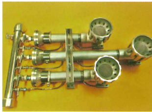
3 連式ライジン LBバーナー
